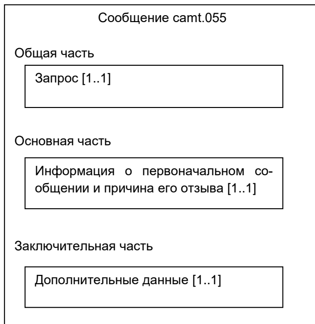
Рисунок 5.1 – Структура сообщения camt.055
