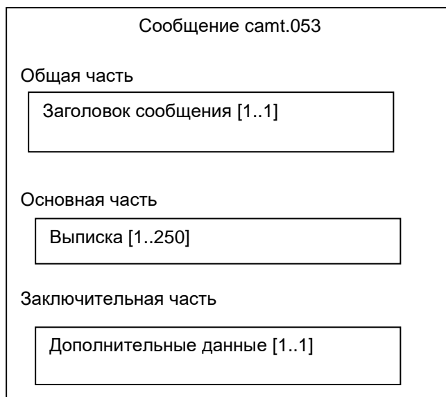
Рисунок 5.1 – Структура сообщения camt.053
